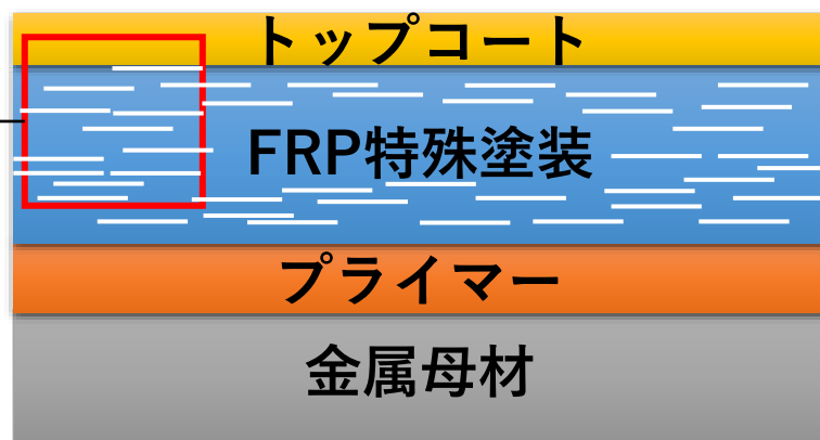
FRP特殊塗装を用いた構成概要
